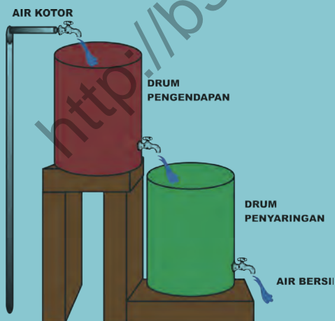
(Sumber: Dokumen Kemdikbud) Gambar 2.13 Cara kerja penyaring air sederhana
