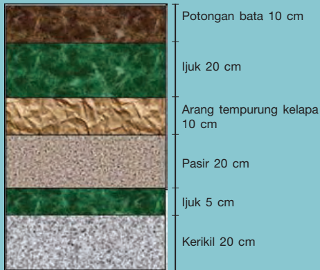
(Sumber: Dokumen Kemdikbud) Gambar 2.12 Blok urutan isi drum penyaring
