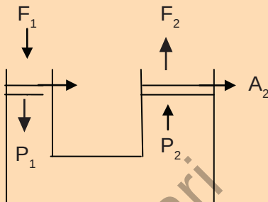
Gambar 7.6 Pompa Hidrolik
